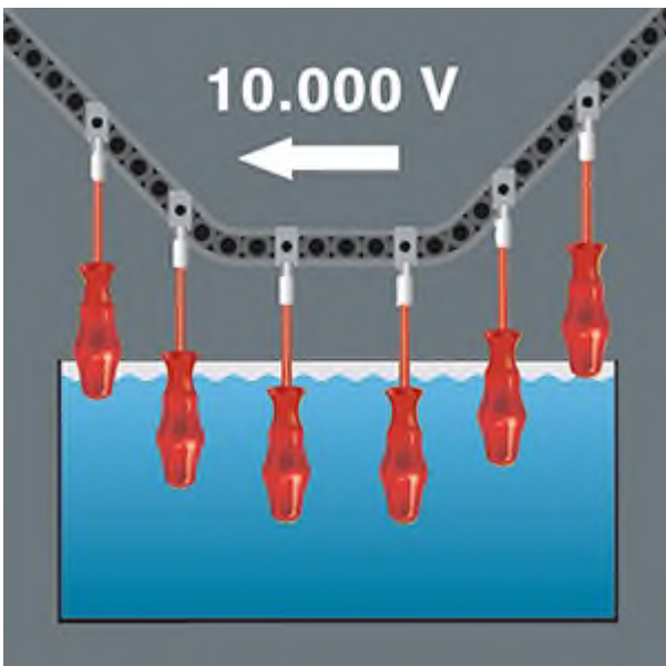
Контроль изоляции
